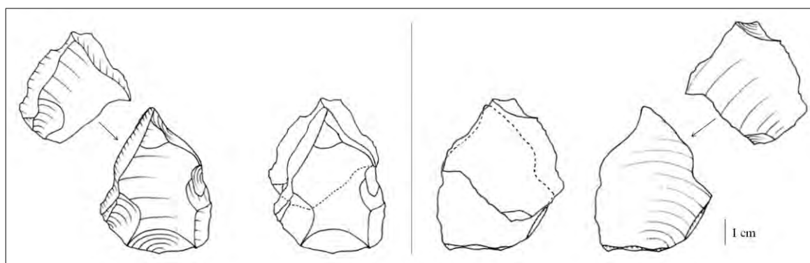
Fig. 8.4.4.4 – Guado San Nicola, US B*C: débitage discoide: [1] scheggia discoide; [2] nucleo discoide (disegni B. Muttillo).
