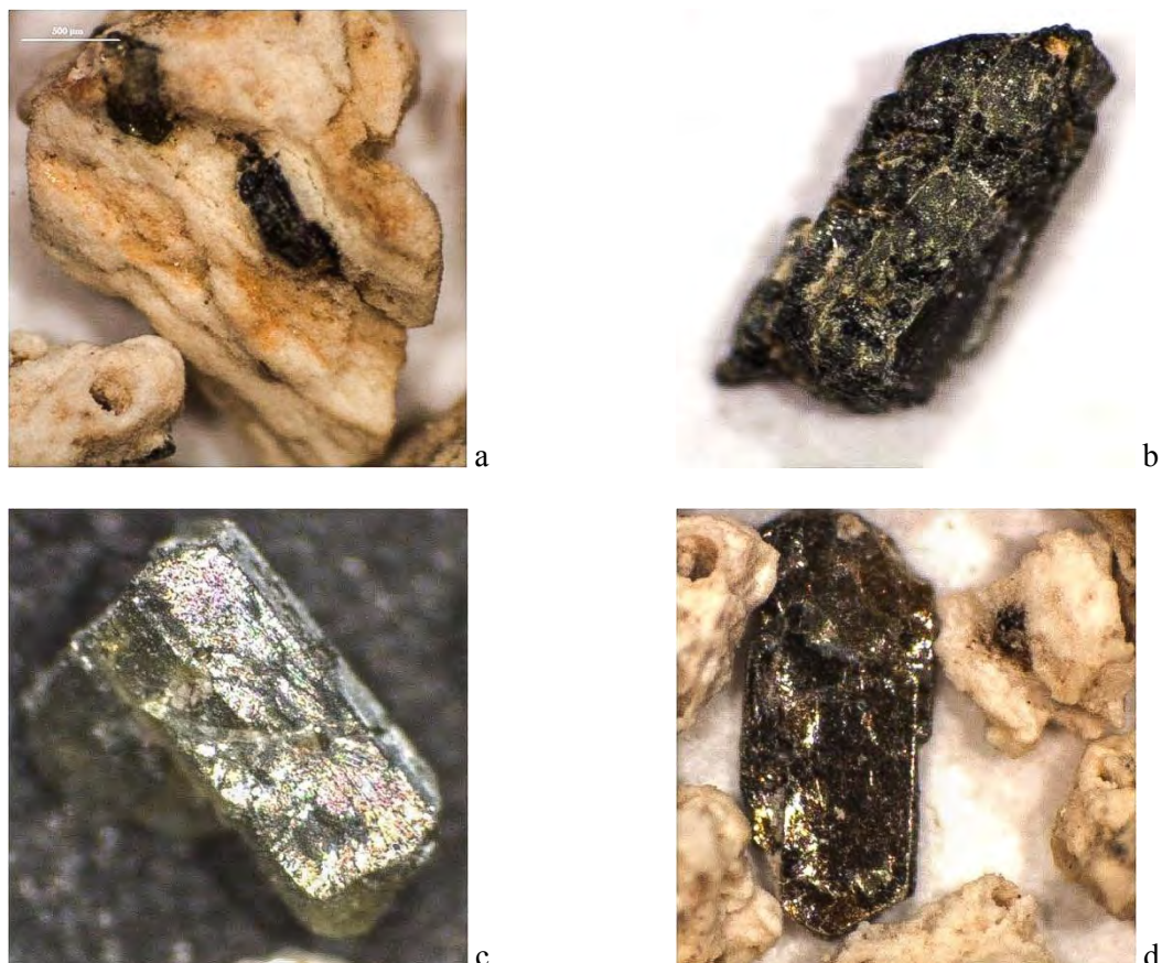
Fig. 3.1.18 - Guado San Nicola: US Tufi. Minerali femici idiomorfi: a) granulo scoriaceo di composizione carbonatica che include cristalli di biotite isorientati parallelamente all'allungamento dei vacuoli, b) cristallo idiomorfo di pirosseno, c) cristallo idiomorfo di anfibolo verde, d) megacristallo di biotite (foto E. Marrocchino).
