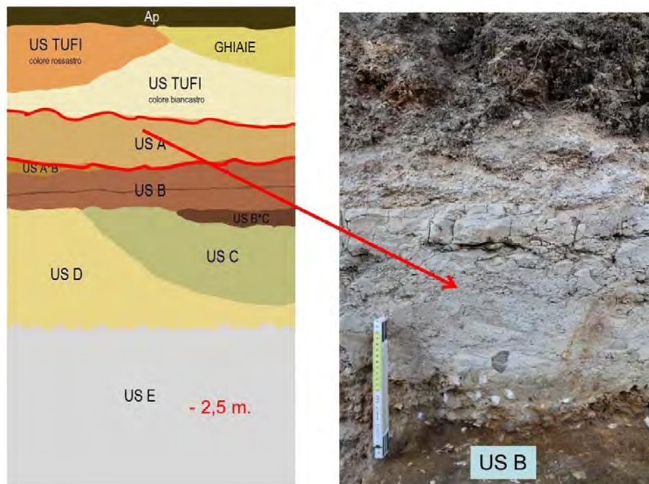
Fig. 3.1.12 - Guado San Nicola: US A. Si tratta di una colata di terra ( earth flow ) con rari ciottoli di litologia varia (foto C. Peretto).
