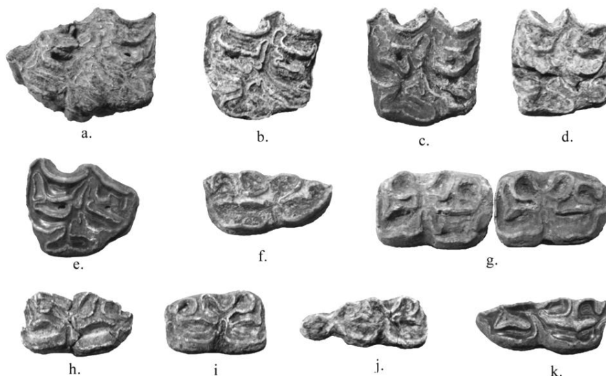
Fig. 7.1.2 - Guado San Nicola. Equus ferus , Denti, veduta occlusale. a: P 2 sx, P09.B*C.33; b: P 3 sx, AV14.B.33; c: P 4 , I13.B.116; dx: M 1 sx, AV14.B.73; e: M 3 sx, P11.B*C.16; f: P 2 dx, P9.B*C.7; sx Mandibola con P 3 -P 4 , R9.C.25; h: M 1-2 , P9.B*C.13; i: M 1 dx, AR14.B.1; j: M 3 dx: P10.B*C.20; k: D 2 sx, R10.B.256 (foto N. Boulbes).
